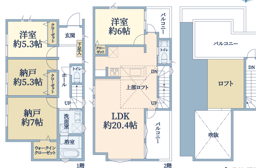
【1号棟 間取図】
